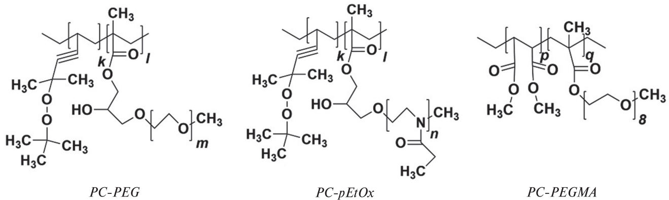
Рис. 1. Структура полімерних наноносіїв полі(ВЕР-ГМА)-графт-мПЕГ (PC-PEG), полі(ВЕР-ГМА)-графт-пЕтОх (PC-pEtOx) та полі(ПЕГМА-ко-ДММ)
